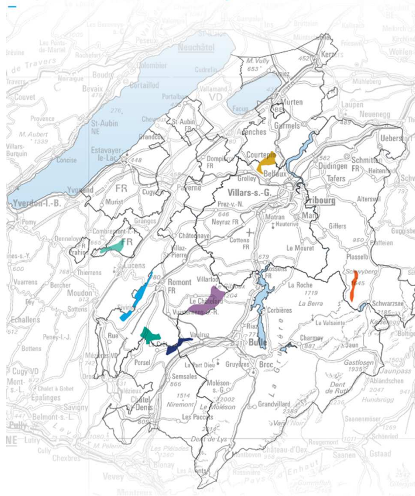
Sites potentiels pour l'exploitation d'énergie éolienne
